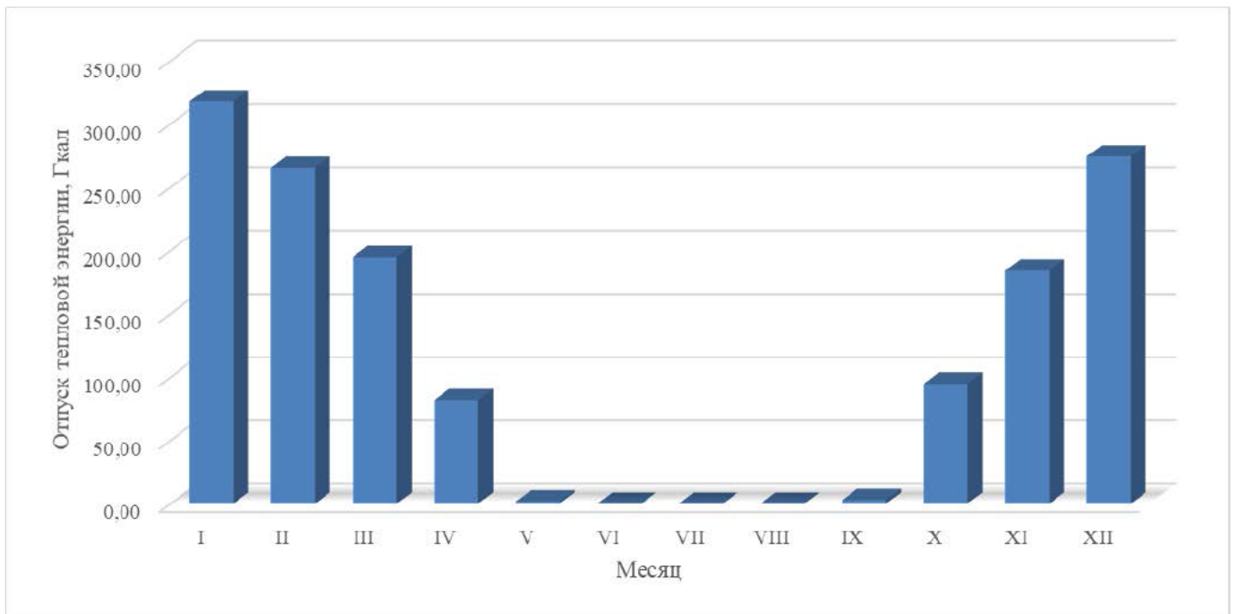
Рисунок 1.2 – Оптимальный температурный график отпуски тепловой энергии для котельной с. Неверовка
