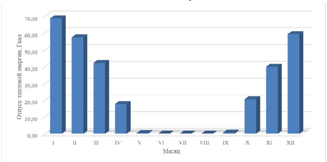
Рисунок 1.3 – Оптимальный температурный график отпуски тепловой энергии для котельной а. Коянбай
